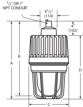
Pendant
